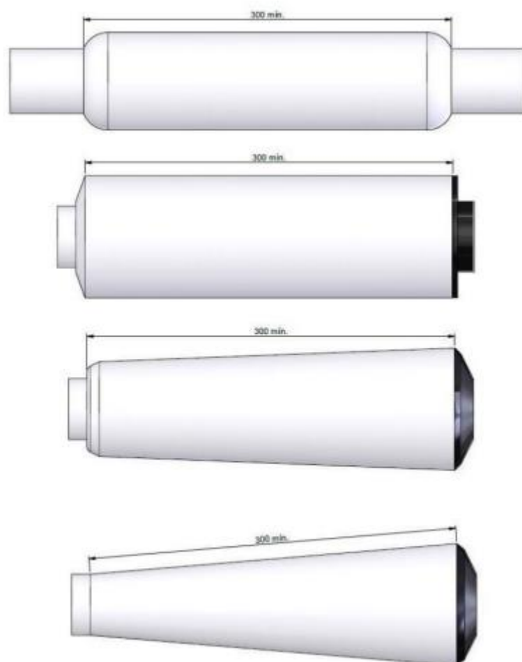
Imagem 10 - Método de medição do abafador.
