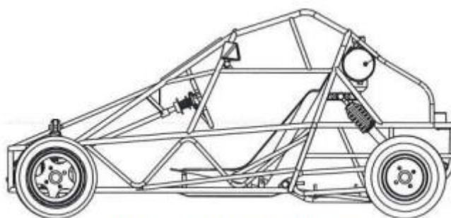
Imagem 1- Modelo de chassi.
